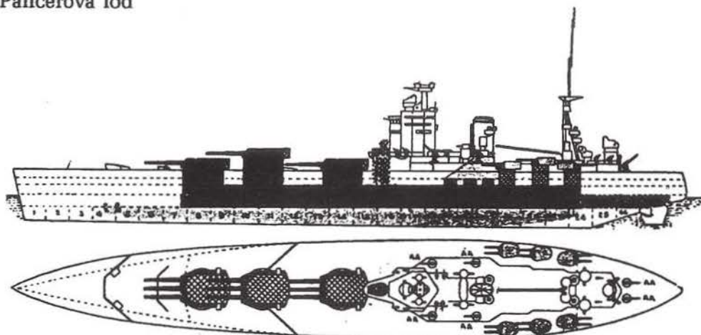
Obr. 4. Angl. bitevní loď „Nelson“. Délka 216 m, šířka 32 m, ponor 9 m, únosnost 40000 t. 9 děl 40 cm, 12 děl 15 cm, 6 děl 12 cm, 12 kulometů proti letadlům.
