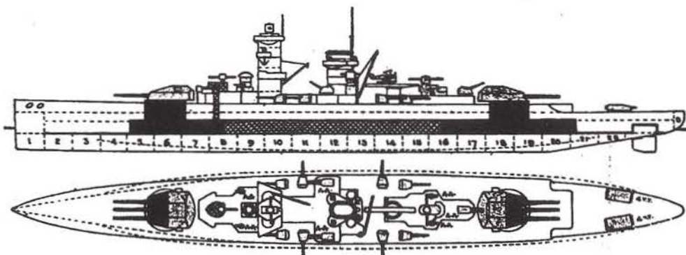
Obr. 6. Něm. bitevní loď „Deutschland“. Délka 186 m, šířka 20 m, ponor 6 m, únosnost 10200 t. 6 děl 28 cm, 8 děl 15 cm, 12 kulometů proti letadlům.
