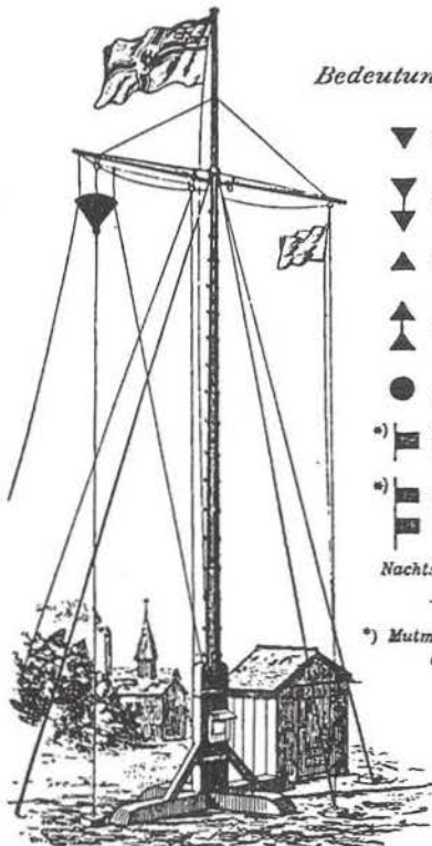
6. Sturmsignalmast der Deutschen Seewarte. (Signal: Sturm aus Südwest; Wind demnächst aus W., NW. u. s. w.)
