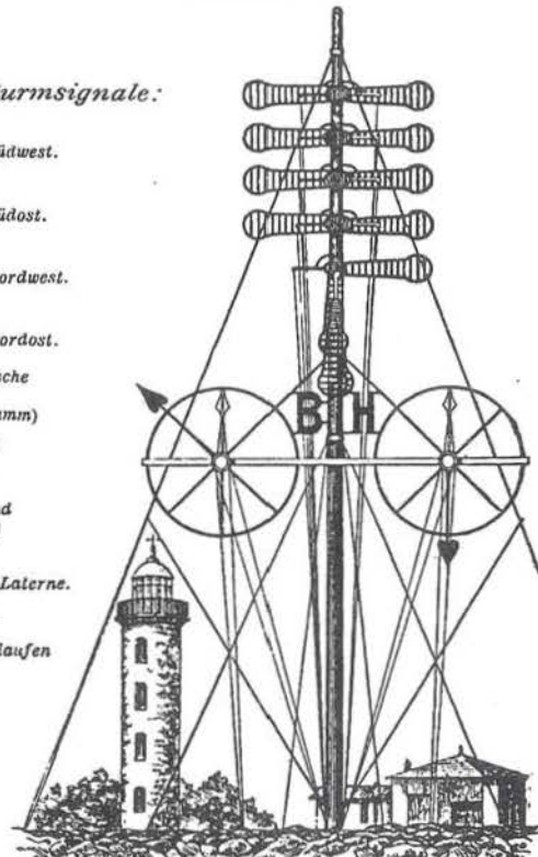
7. Windsemaphor an der Nordseeküste. (Signal: Borkum mäfsiger NW., Helgoland frischer S.)
