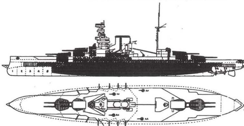
Obr. 5. Angl. bitevní loď „Queen Elisabeth“. Délka 195 m, šířka 31 m, ponor 10 m, únosnost 33500 t. 8 děl 38 cm, 12 děl 15 cm, 6 kulometů proti letadlům.
